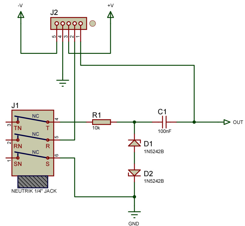
ML12.DI1 - Passive DI input circuit.
