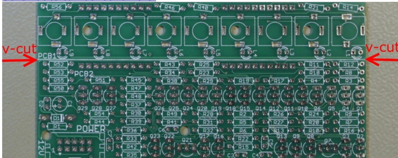
Empty PCB.
