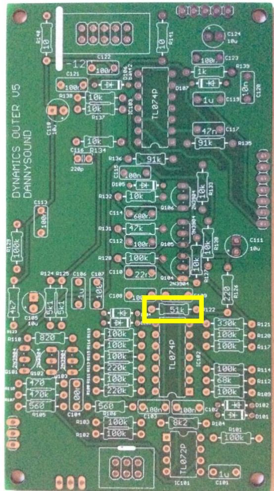
12) – 1 x 51k (R122)
