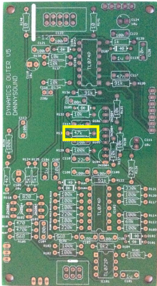
11) – 1 x 47k (R131)
