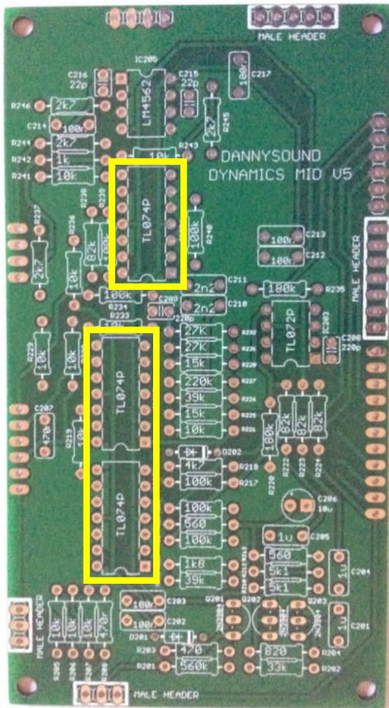
59) – 3 x 14 Pin Socket (IC201, IC202, IC204)
