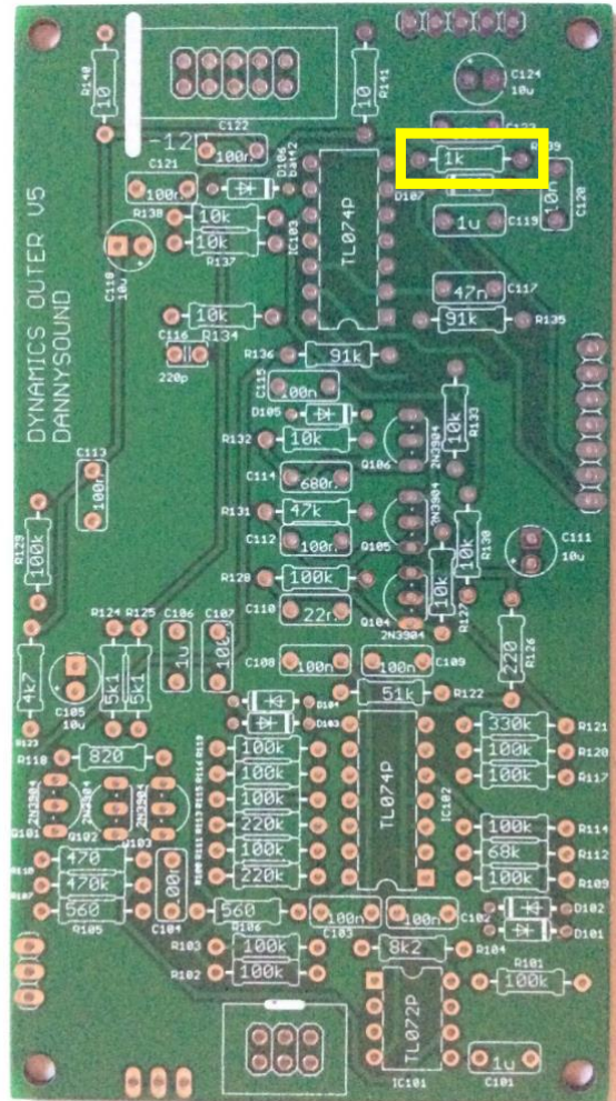
6) – 1 x 1k (R139)
