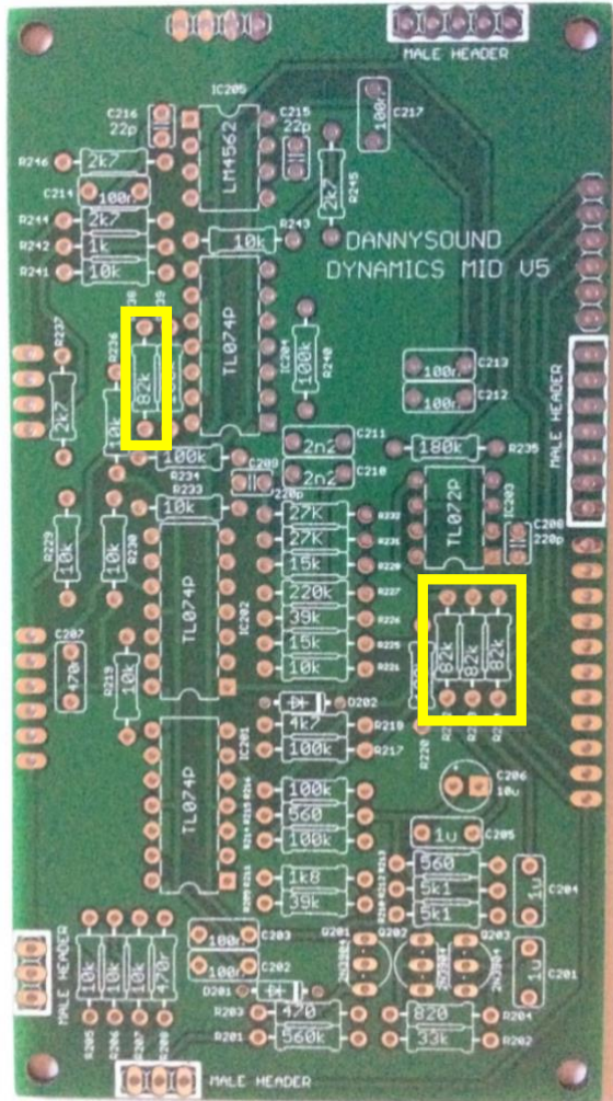
52) – 4 x 82k (R222, R223, R224, R238)
