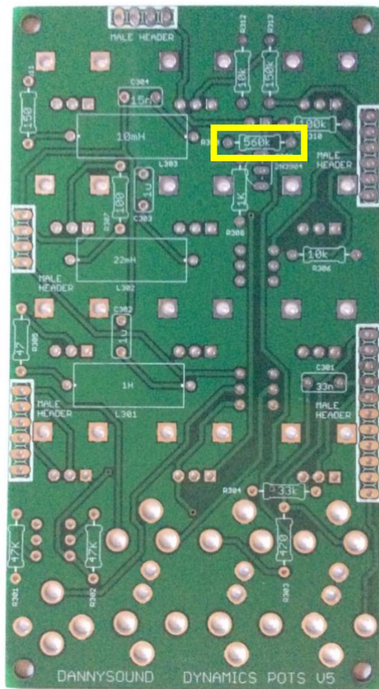
88) – 1 x 560k (R309)
