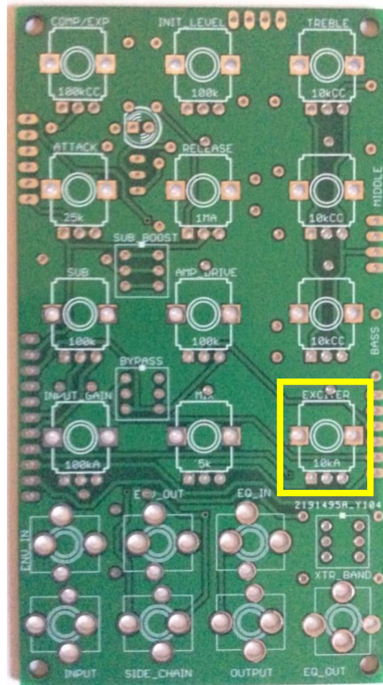
107) – 1 x A10K ALPHA POT (Metal, green)
