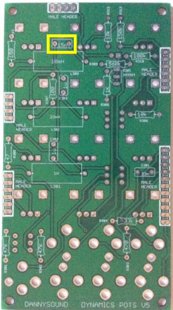
89) – 1 x 15n film (C304)
