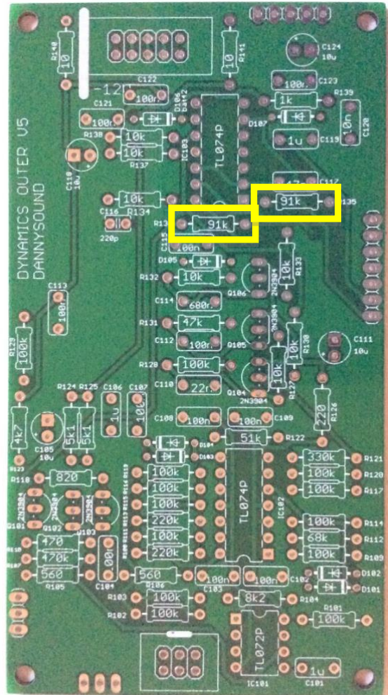
14) – 2 x 91k (R135, R136)
