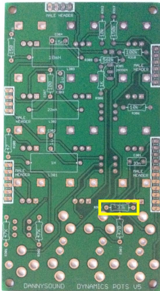
84) – 1 x 33k(R304)
