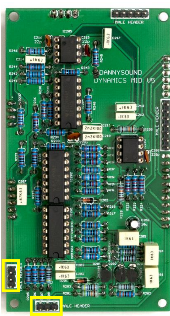
69) – 2 x 3 Pin MALE header
