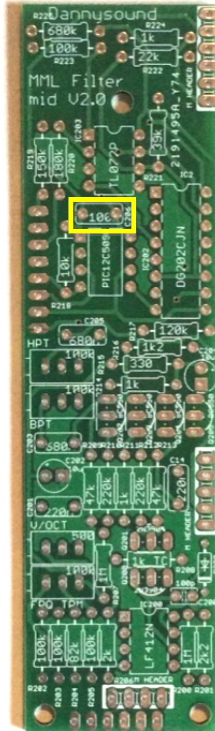
55) – 1 x 100n box (C208)
