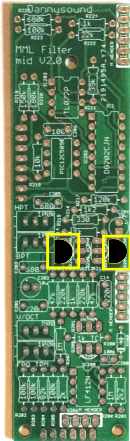
59) – BC550 MATCHED PAIR (Q202, Q205)
