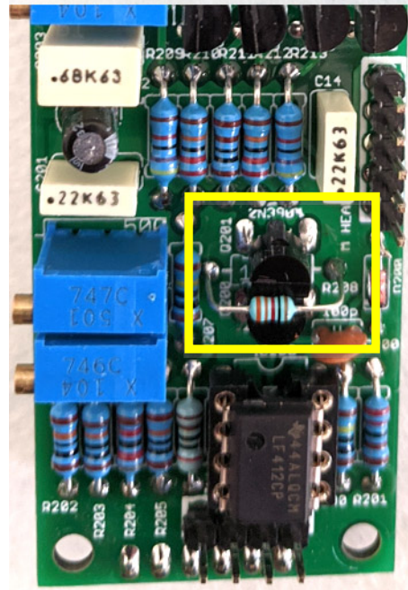
62) – 1 x 1k Tempco (R208)
