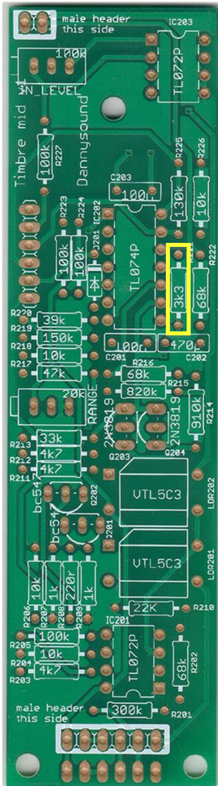
27 - 1 X 3k3 (R221)
