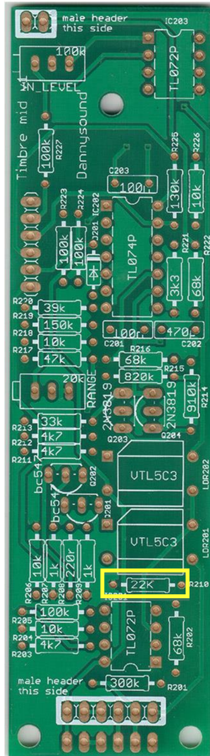
30 - 1 x 22k (R210)
